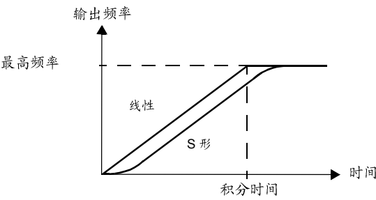
图 42 定义加减速积分时间曲线
