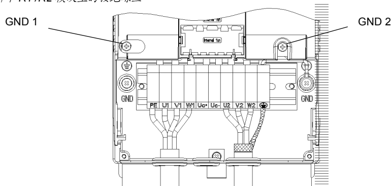
图 16 拆下 R3/R4 模块上的接地螺丝
