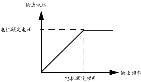
图 36 输出电压与输出频率的关系
