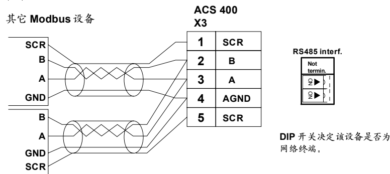
图 29 I/O 示例
