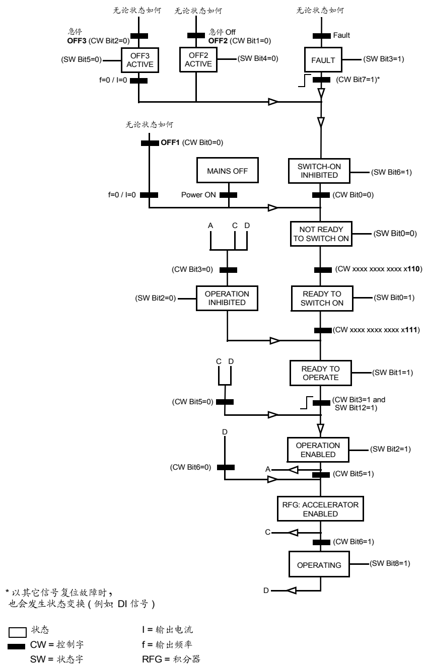
图 69 启动和停止信号的状态评价示意图
