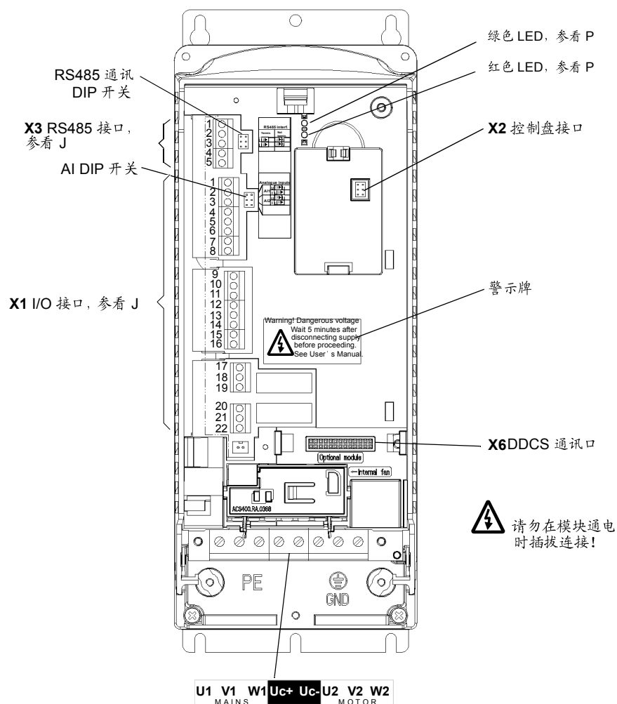
图 11 接口和端子
